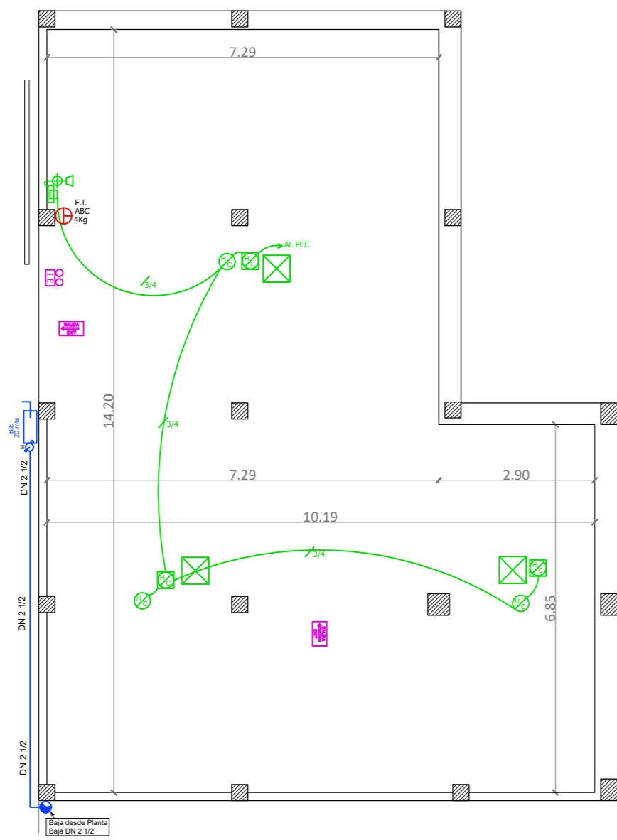
PLANTA DEPÓSITO ESC.: 1/100
