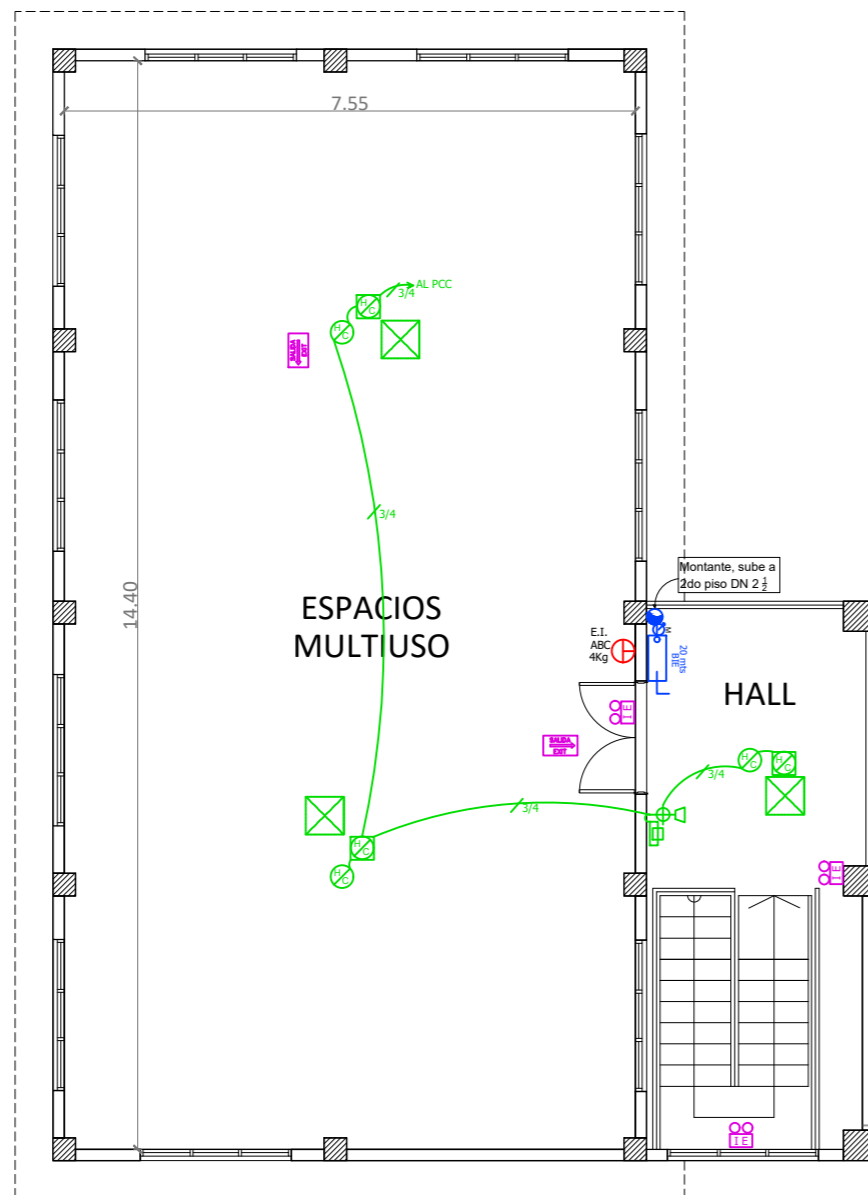
PLANTA 1º NIVEL ESC.: 1/100
